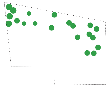
laag 4: bomen
