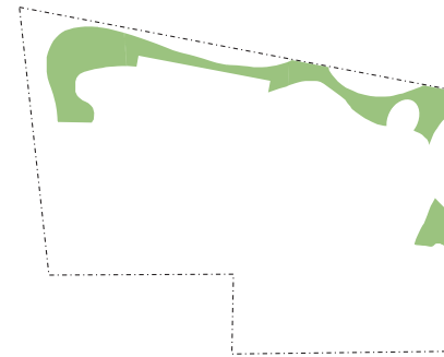
laag 2: meerjarigen
